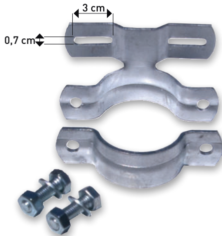
Rohrschelle 70 mm Lochabstand
