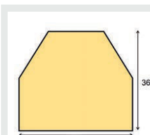
Flächenschutz Trapez, Typ CC
