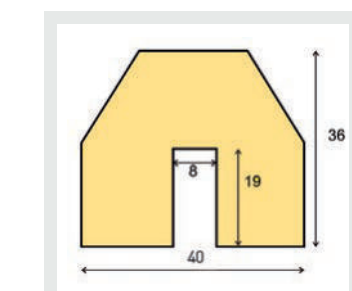
Profilschutz Trapez, Typ BB
