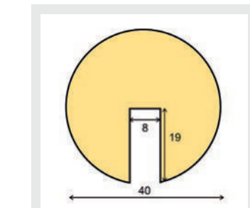
Profilschutz Kreis, Typ B
