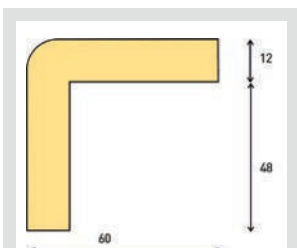
Kantenschutz Winkel, Typ H+
