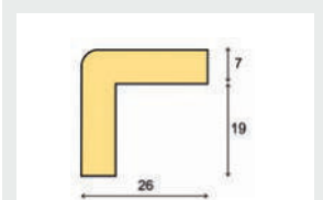
Kantenschutz Winkel, Typ E
