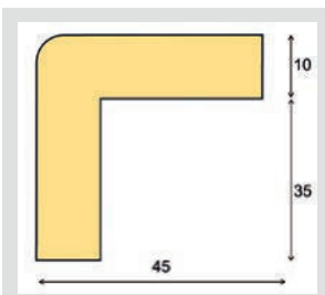
Kantenschutz Winkel, Typ H
