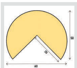
Kantenschutz Kreis, Typ A+
