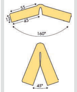
Kantenschutz Flex, Winkel, Typ H+
