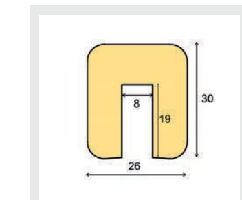
Profilschutz Viereck, Typ G
