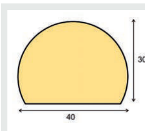
Flächenschutz Kreis, Typ C
